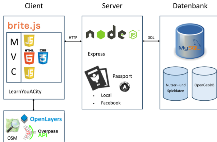
Abb. 4: Client-Server Architektur für das implementierte kartenbasierte Lernspiel
